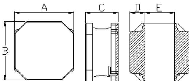
Dimension (Unit:mm)
