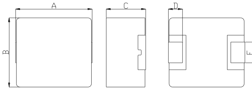
Dimension (Unit:mm)
