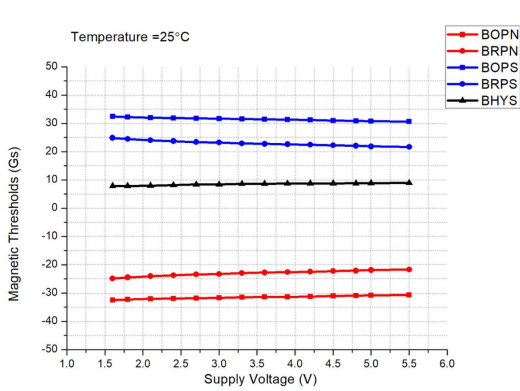
磁场阈值 vs. 供电电压 @TA=25°C
