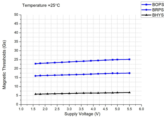
磁场阈值 vs. 供电电压 @TA=25°C
