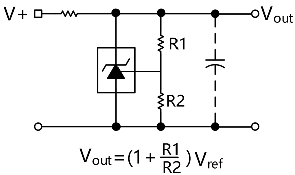
图 18. 并联电压
