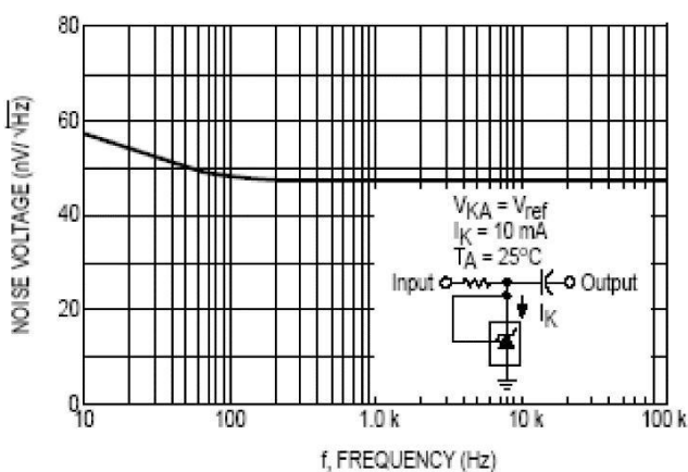
图 13. 光谱噪声密度
