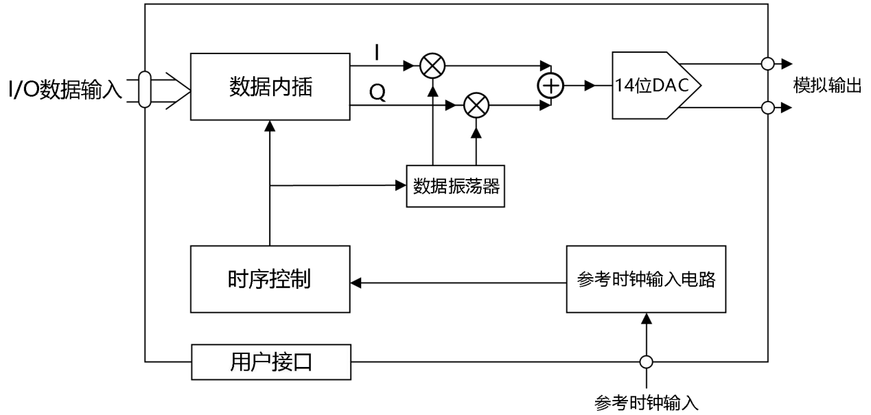
图 1 CBM99D57 功能框图
