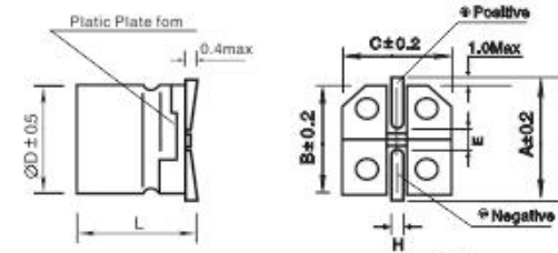
Fig. 2 (≥ Φ12.5)
