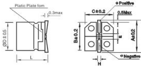
Fig. 1 (Φ4~Φ10)
