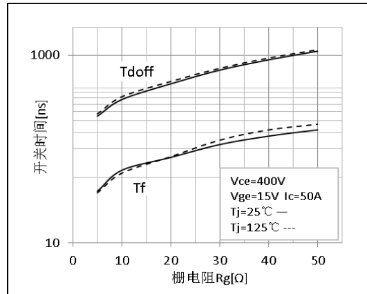
图 8 关断-栅电阻特性曲线
