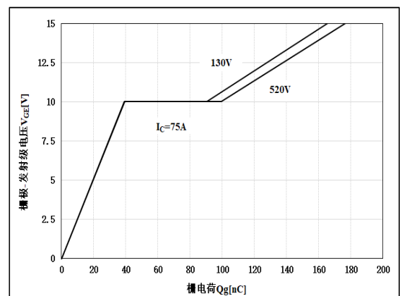
图 18 栅电荷特性
