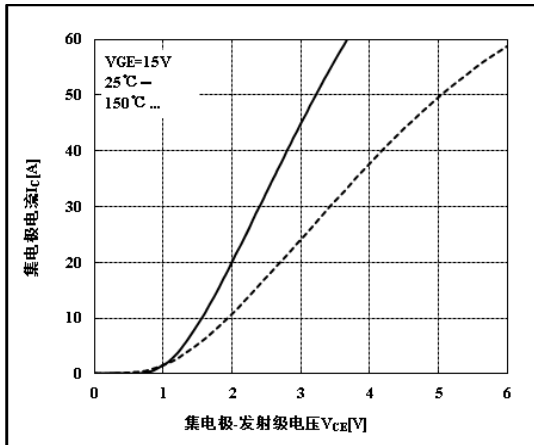
图 3 饱和和压降特性
