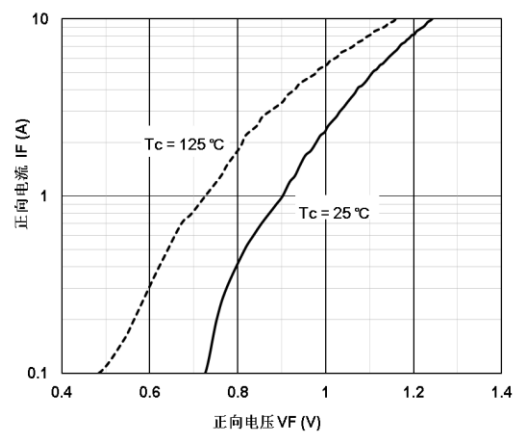
图 12. 二极管的正向压降特性
