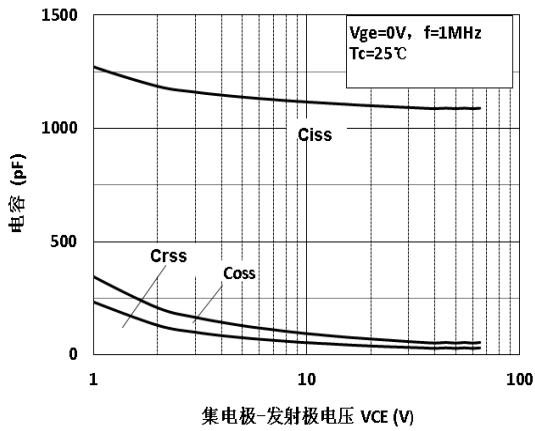
图 13.电容特性
