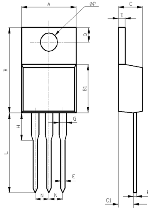
外形图: CRG15T60A83L (TO-220)
