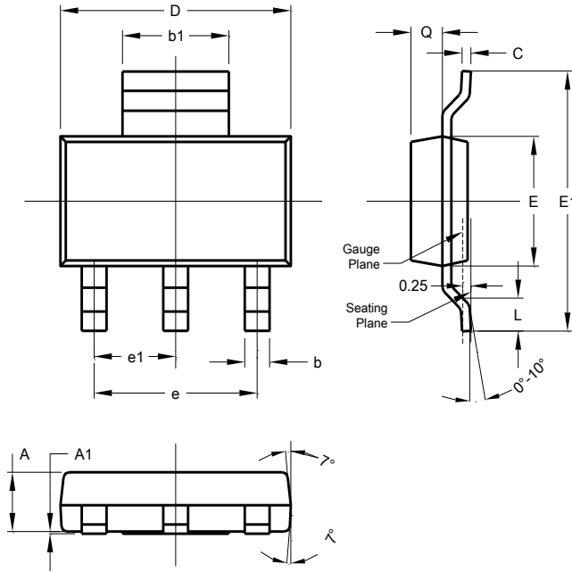
SOT223
