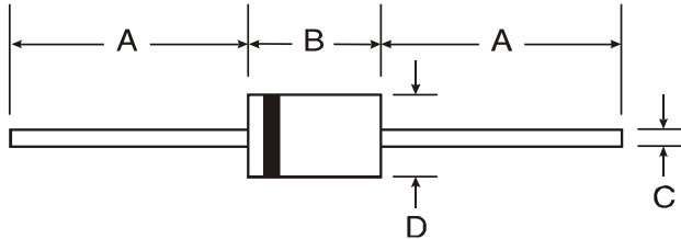
DO-201AD
