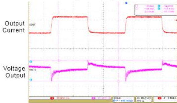
Load Transient I_o=0-500\text{mA} , V_o=3.3\text{V} , V_{in}=5\text{V}
