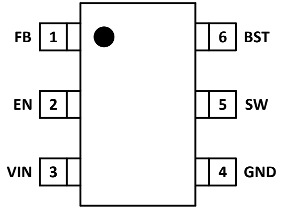
TSOT26
