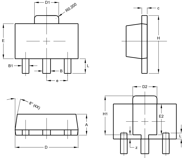
SOT89
