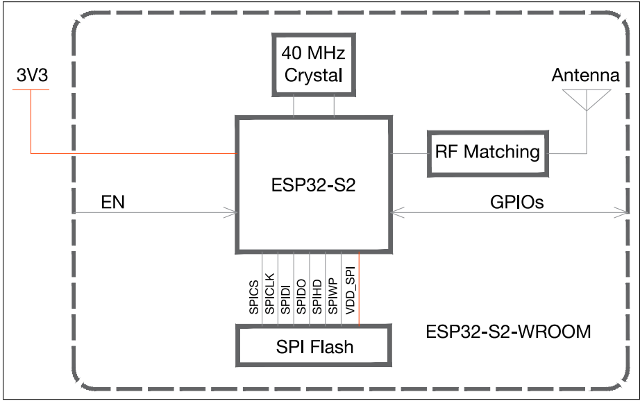
图 1: ESP32-S2-WROOM 功能块图
