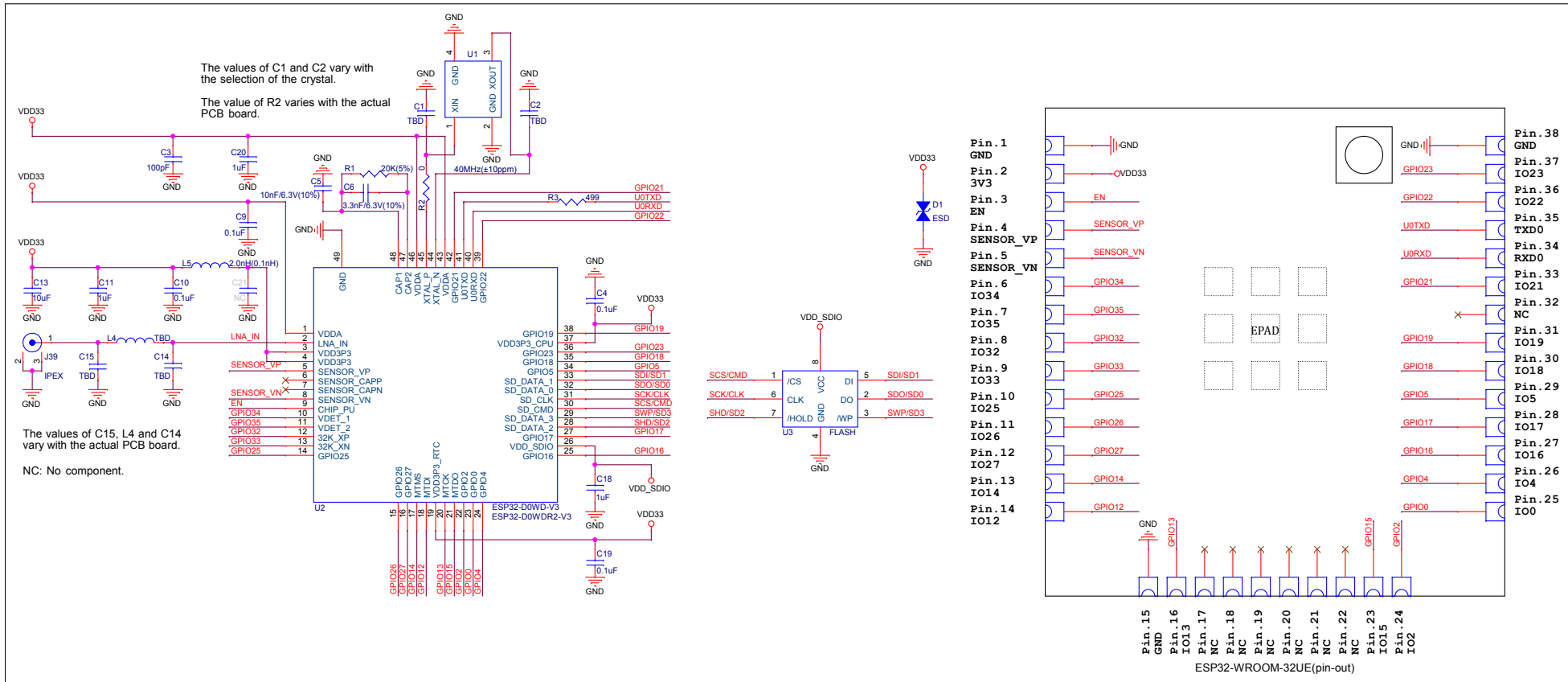
图 7: ESP32-WROOM-32UE 原理图
