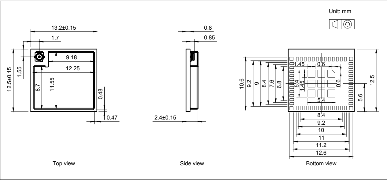
图 9: ESP8684-MINI-1U 尺寸
