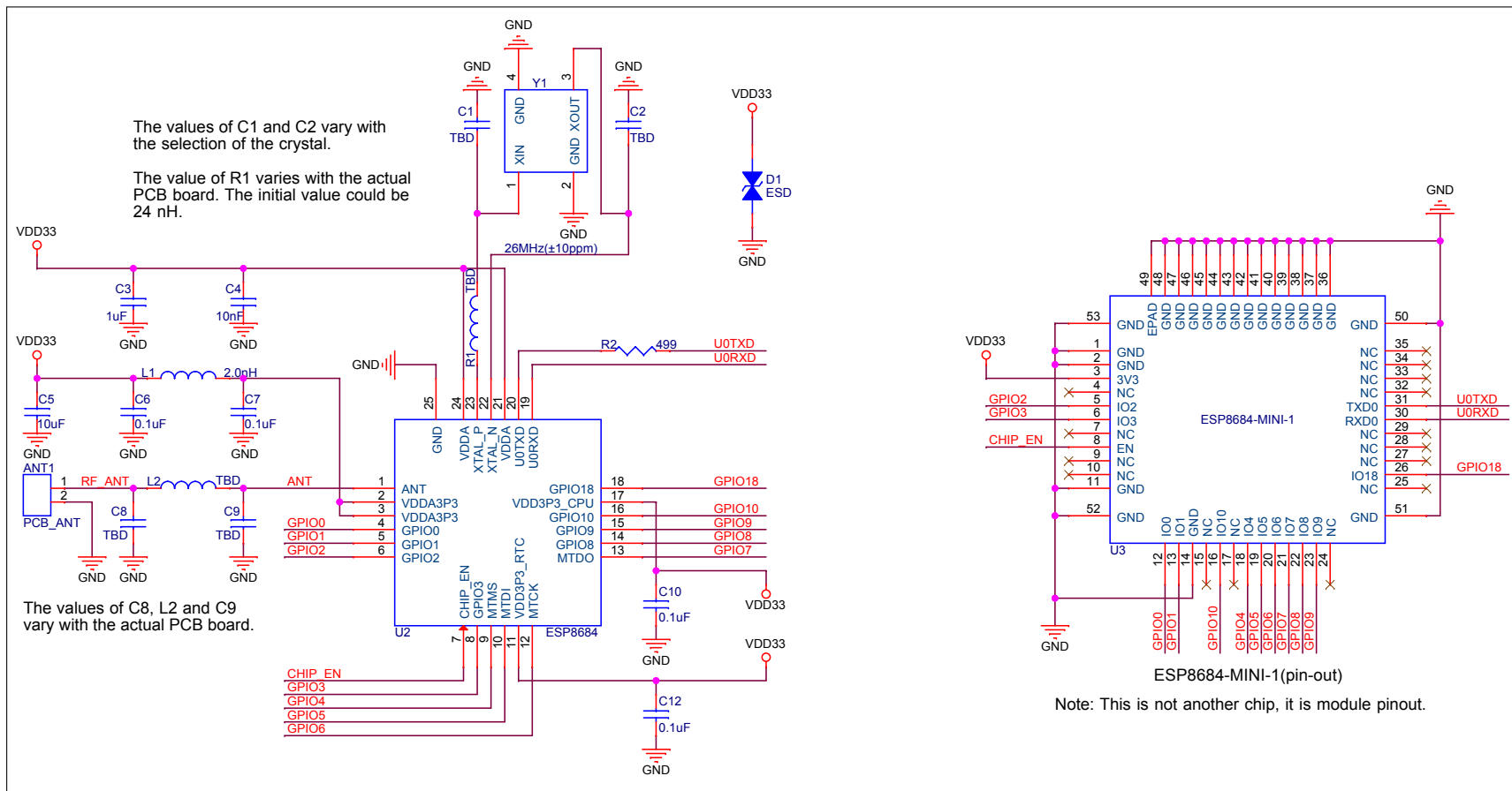
图 5: ESP8684-MINI-1 原理图
