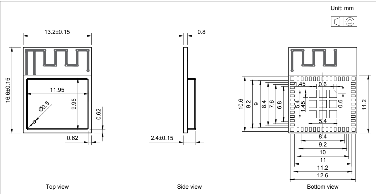
图 8: ESP8684-MINI-1 尺寸
