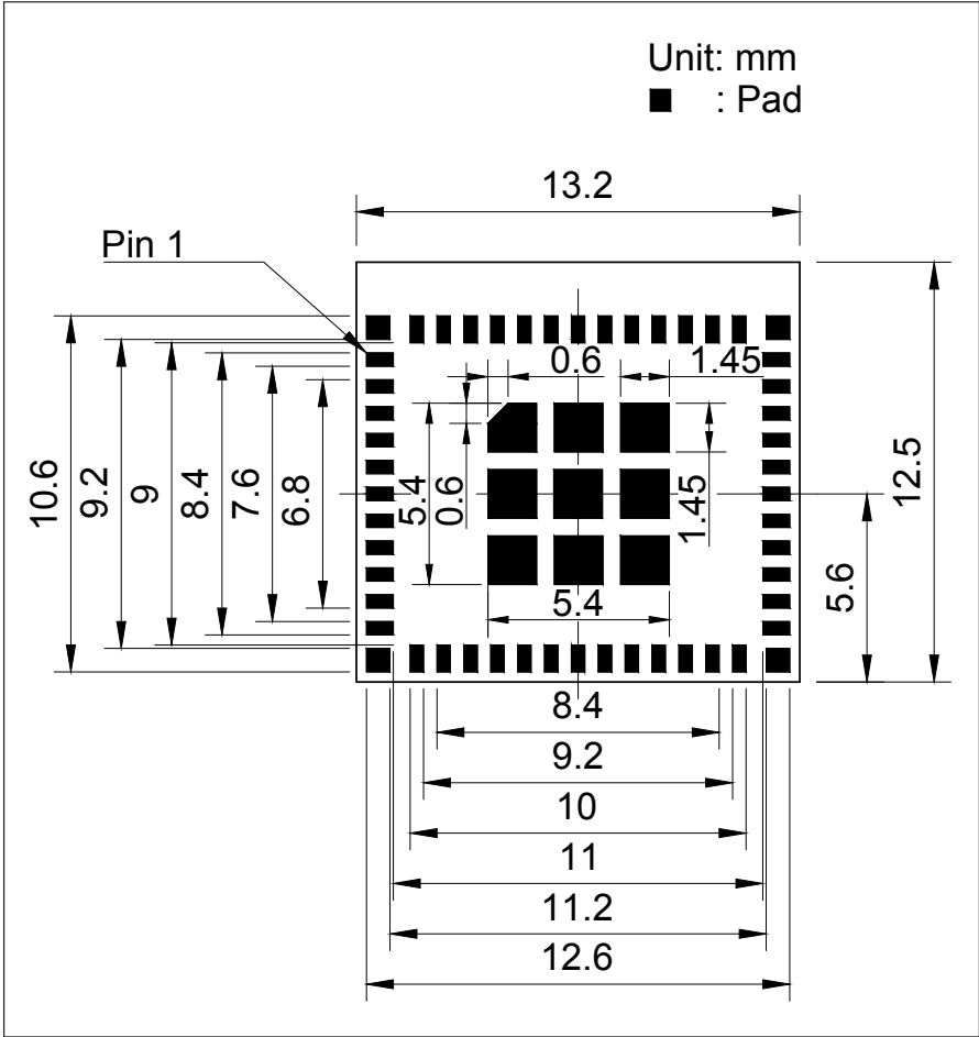
图 11: ESP8684-MINI-1U 推荐 PCB 封装图形
