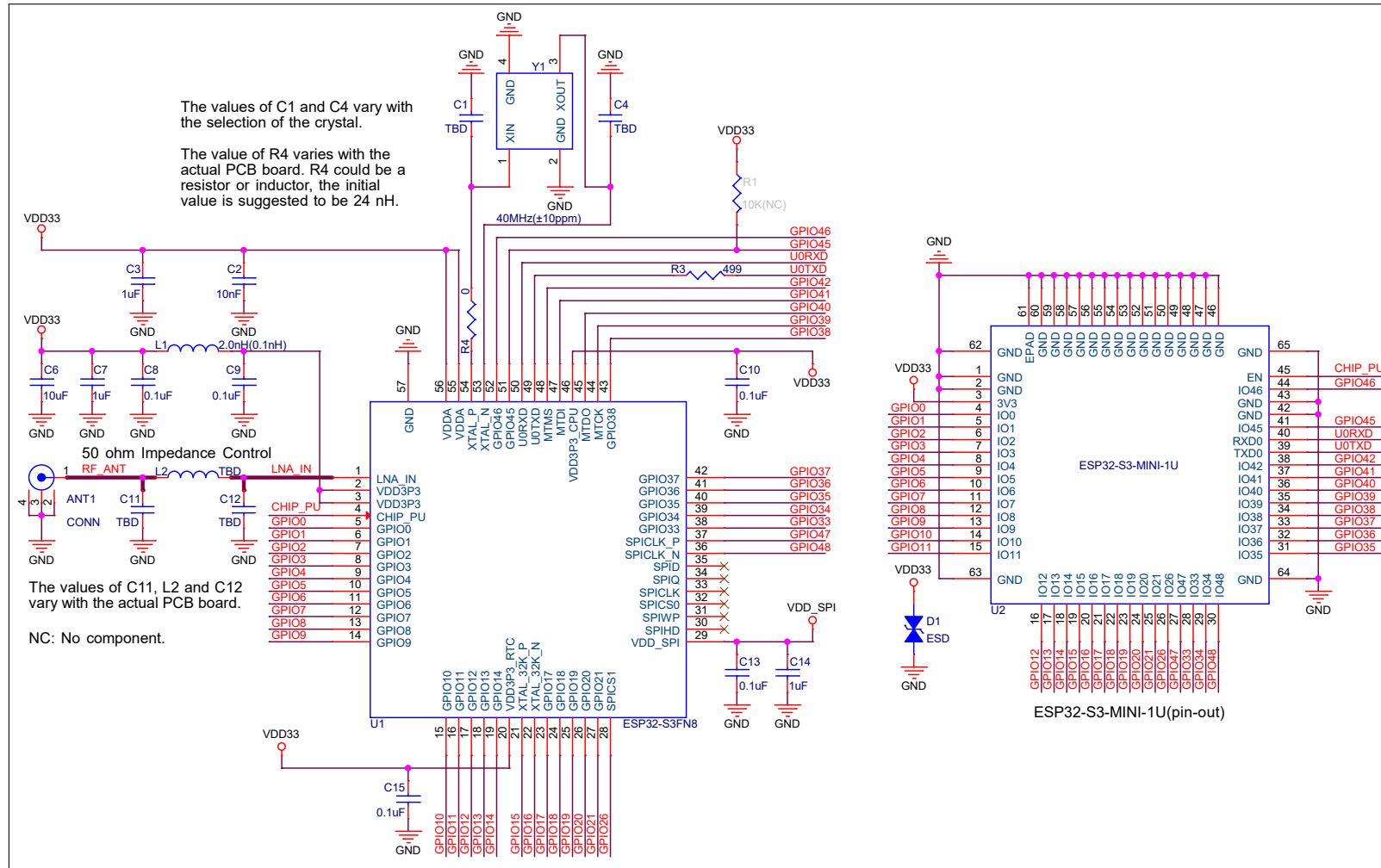
图 6: ESP32-S3-MINI-1U 原理图
