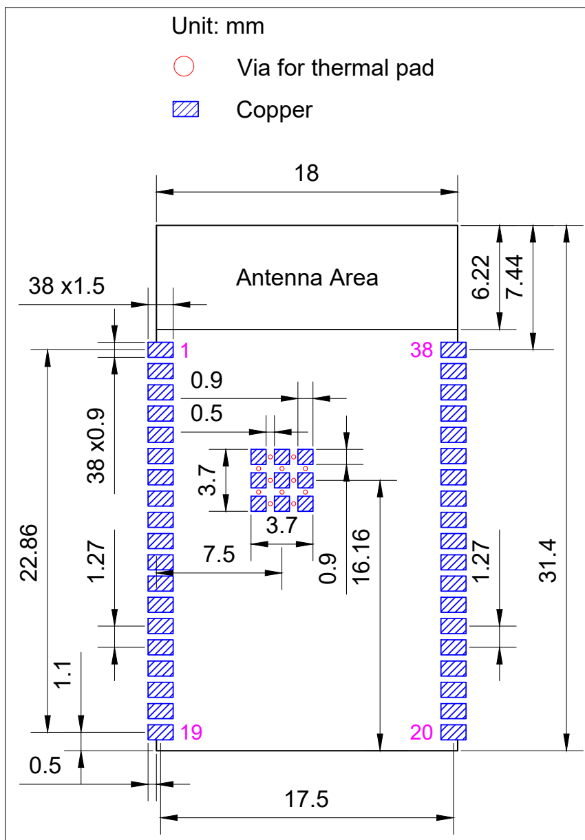
图 12: PCB 封装图形
