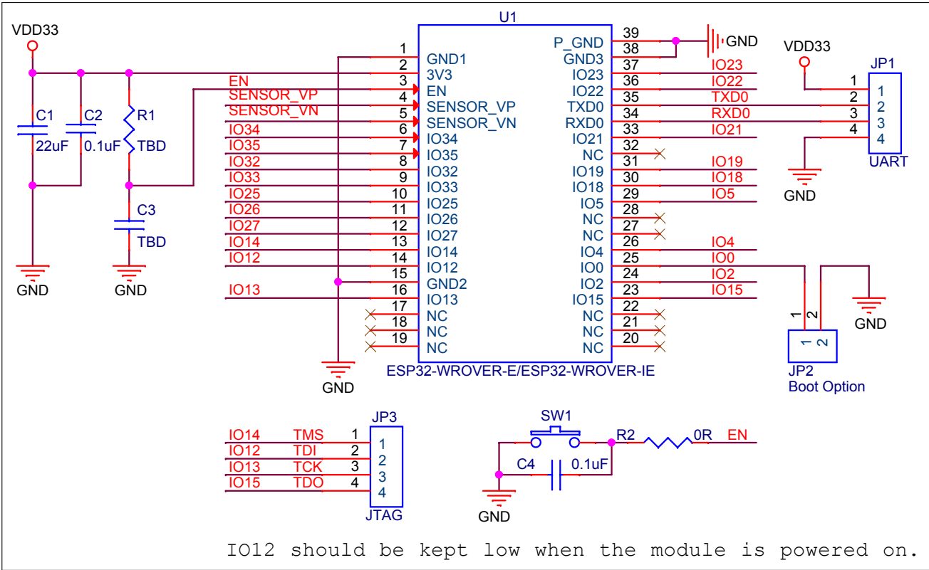
图 7: 外围原理图
