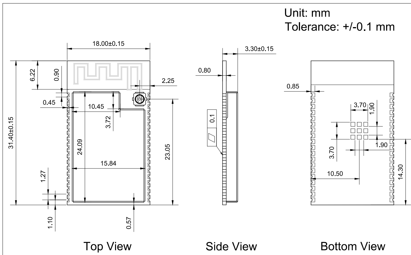
图 10: 模组尺寸图
