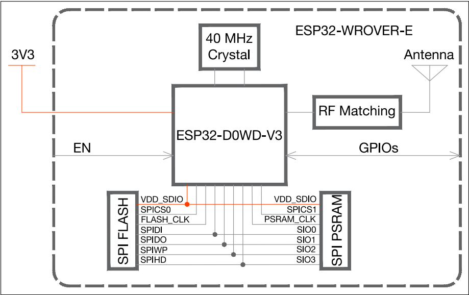
图 1: ESP32-WROVER-E 模组功能块图
