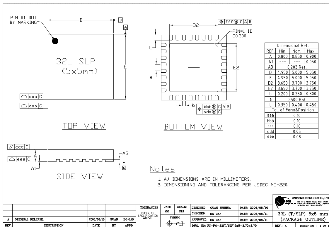
图 6-1. ESP8266EX 封装
