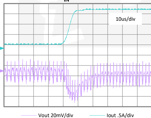
1.2V Load Step rising 0.3A-2A V_{IN}=12\text{V}
