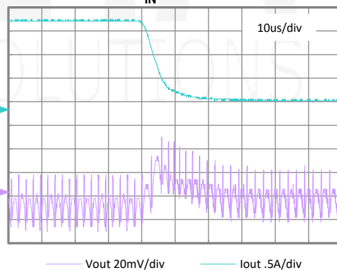
1.2V Load Step falling 2A-0.3A V_{IN}=12\text{V}
