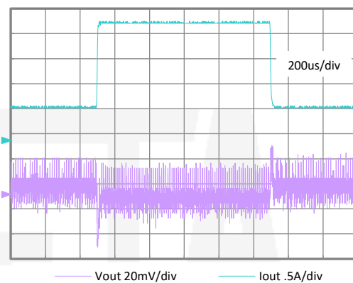
1.2V Load Step 0.3A-2A-0.3A V_{IN}=12\text{V}
