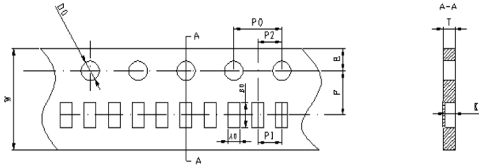
图5 载带适用于0402尺寸规格
