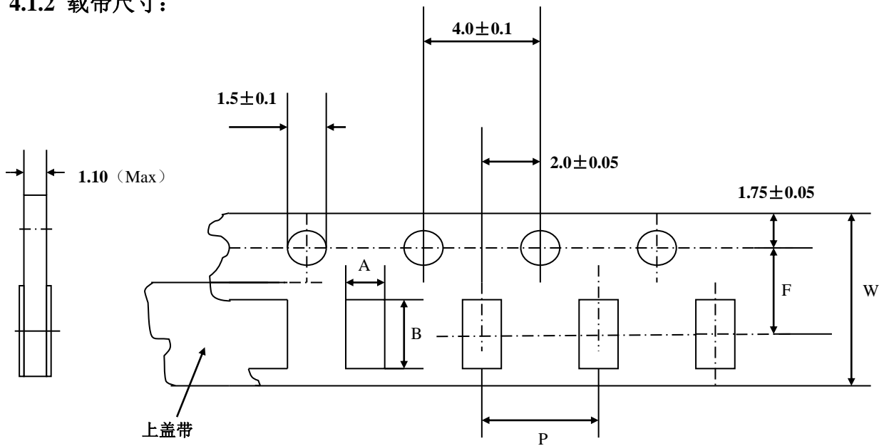
图 2 载带
