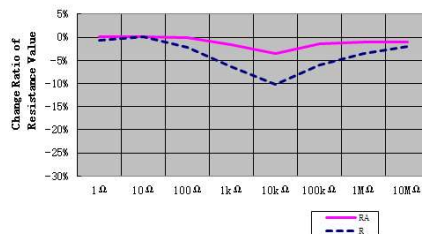
2512size: ±10kV
