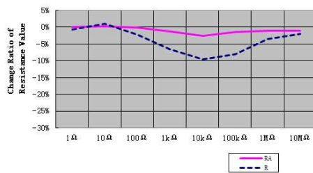
2512size: ±10kV
