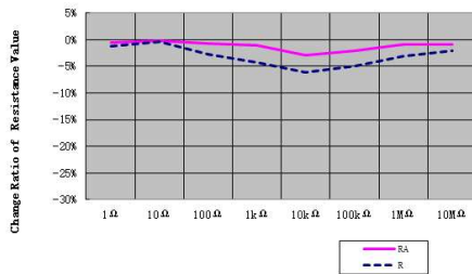
0805size: ±4kV
