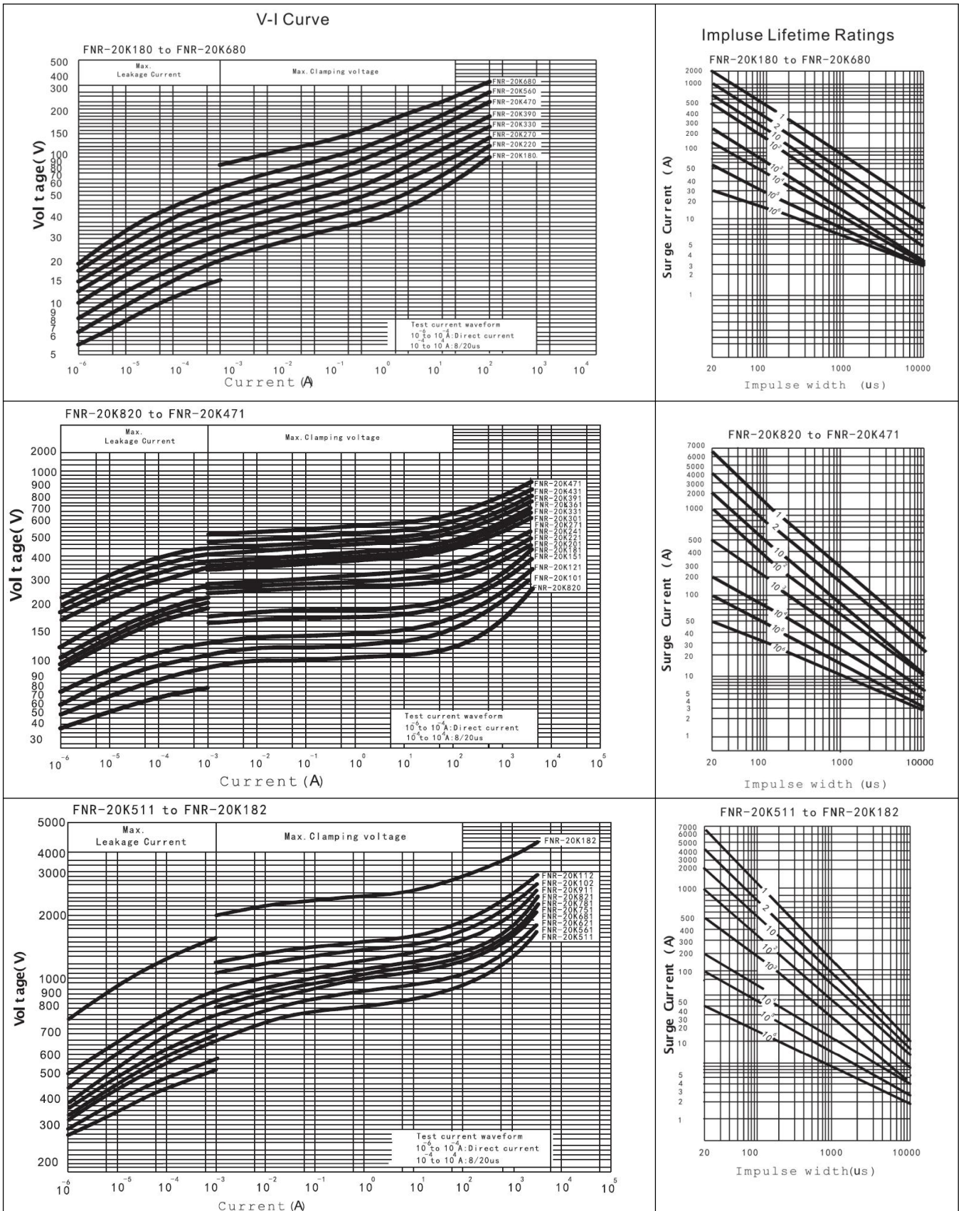
*20K 系列 V-I 特性曲线和最大浪涌电流降额曲线
