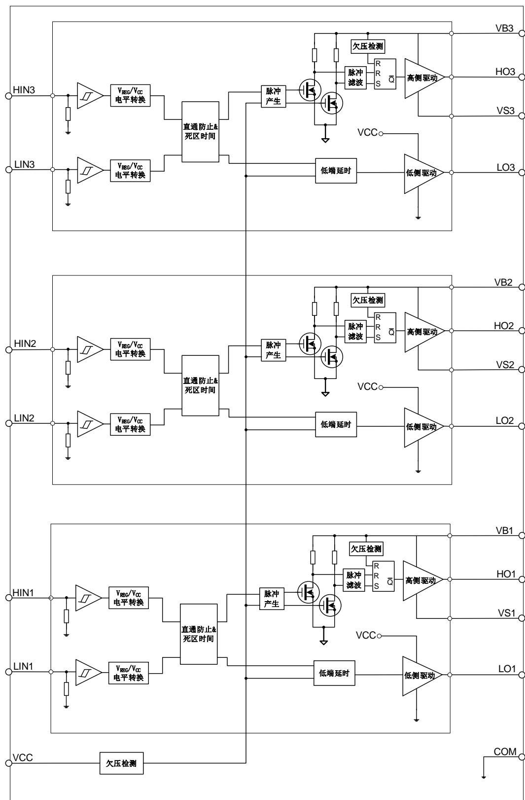
图 1-2 FD6288 功能框图
