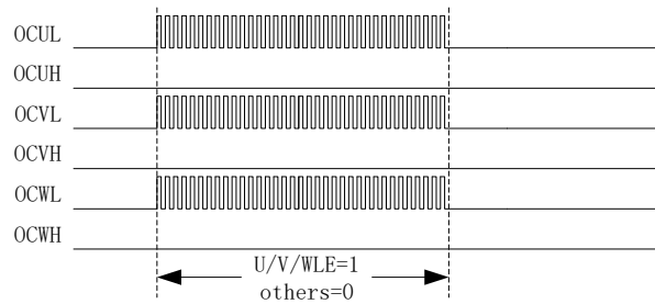
图 18-8 刹车图
