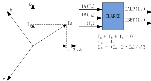
图 14-4 CLARKE 变换
