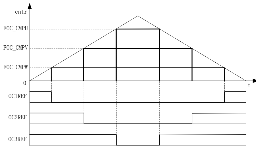
图 19-3 PWM 生成图
