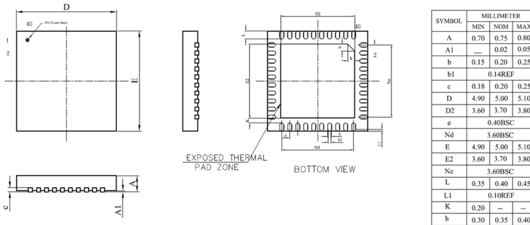
图 3-1 QFN40 5mm X 5mm 封装尺寸图
