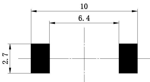
焊接处尺寸图
