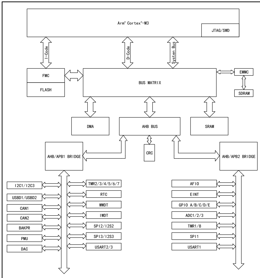
图 6 APM32F103xCTxS (合封 SDRAM) 系统框图
