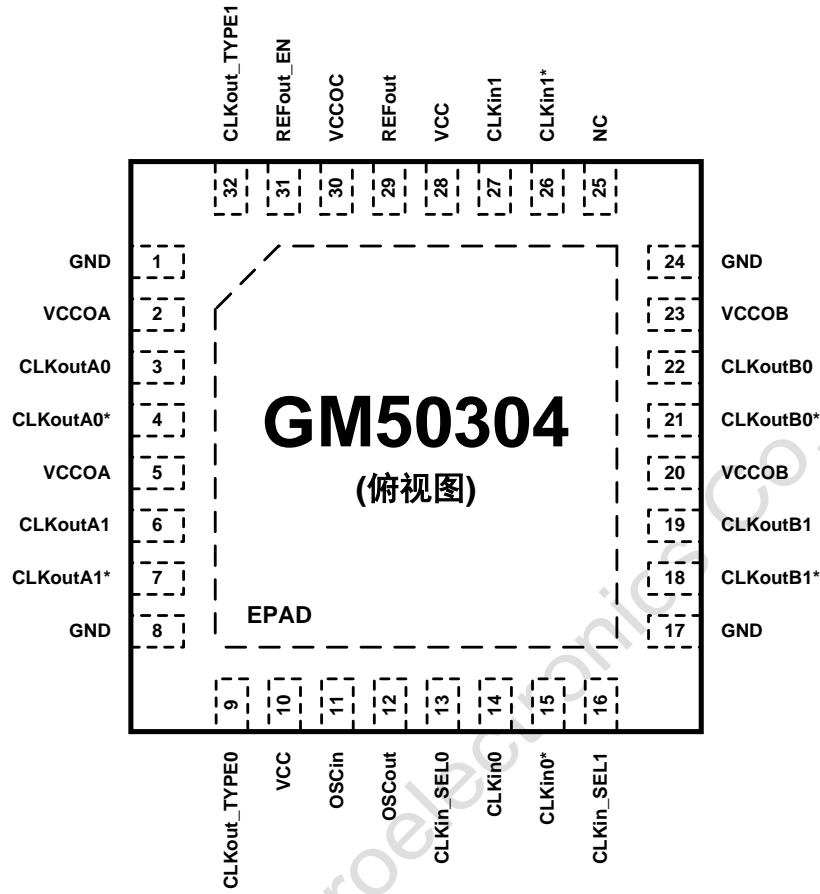
图 2, 引脚配置
