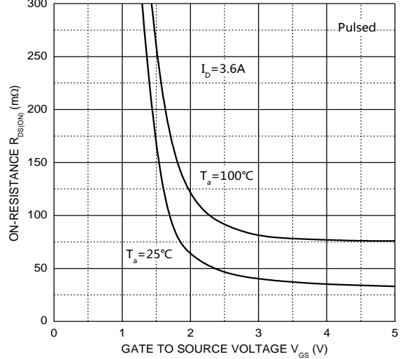
R_{DS(ON)} - V_{GS}
