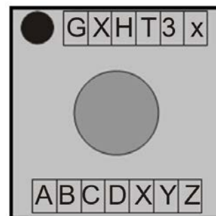
图 13 GXHT3x-DIS 顶视图以及激光标记
