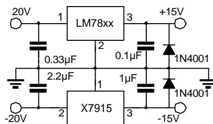
图11 分电源电路(±15V, 1A)
