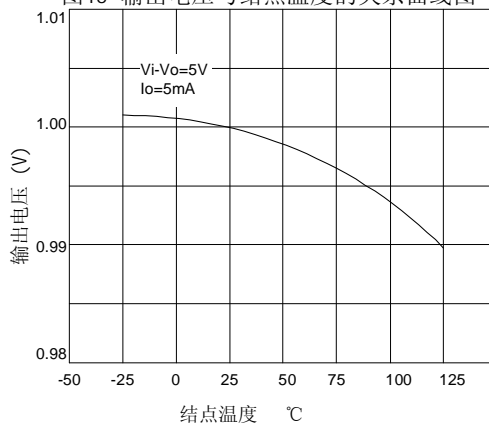
图15 输出电压与结点温度的关系曲线图
