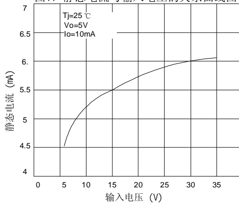
图17 静态电流与输入电压的关系曲线图
