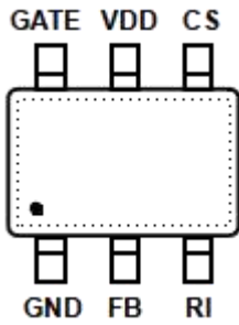
SOT23-6 (顶视图)
