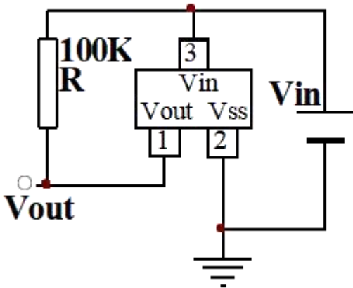
N-ch Open Drain 输出
