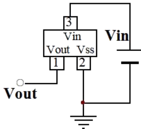
CMOS 输出
