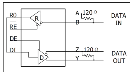
图 11. HX3080E/ HX3083E/ HX3086E 全双工模式下的中继器
