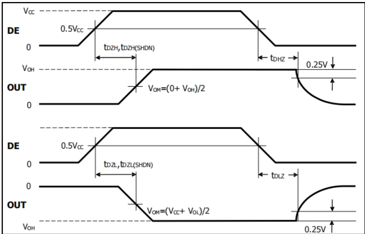
图 6.驱动器使能和禁用时序( t_{DZH} 、 t_{DZH(SHDN)} 、 t_{DZH} 、 t_{DZL} 、 t_{DZL} 、 t_{DZL(SHDN)} )
