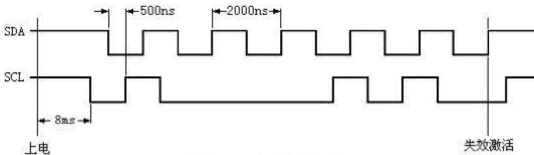
图 9.POR 失效时序图
