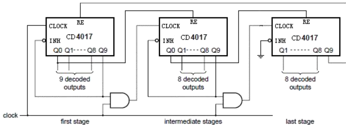
图 10 扩展计数器
