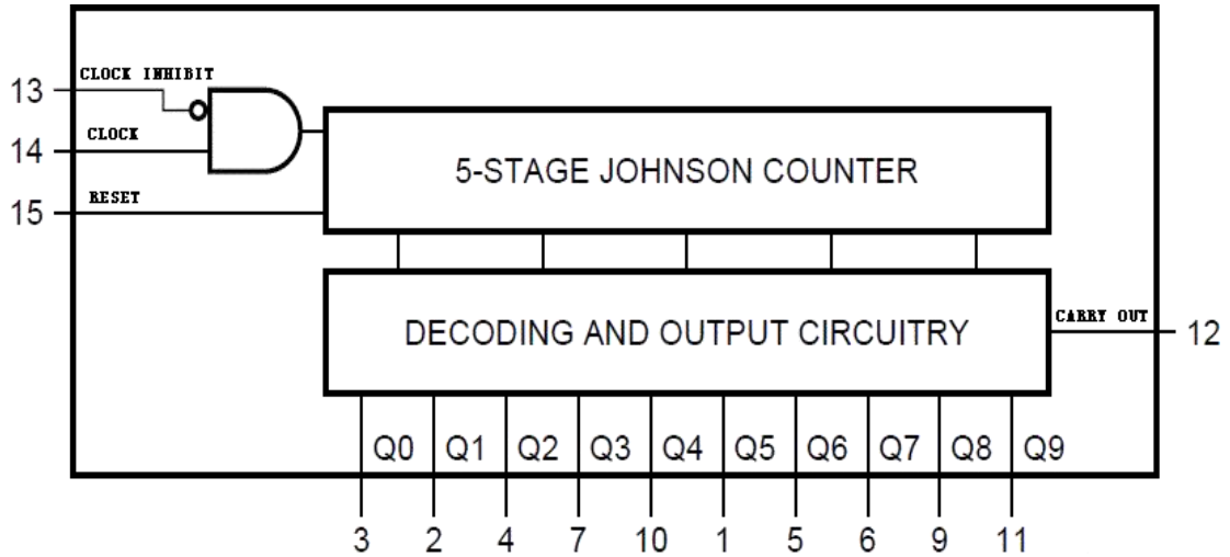
图 1 功能框图
