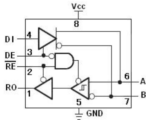
图2: SN75176 逻辑图
