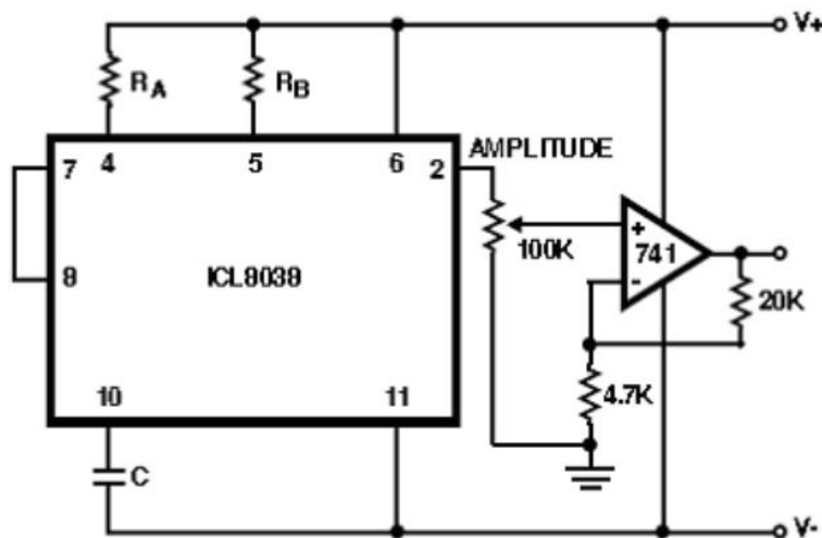
图 6.正弦波输出端缓冲放大器
