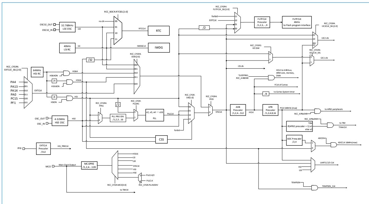
图 3-4 时钟树
