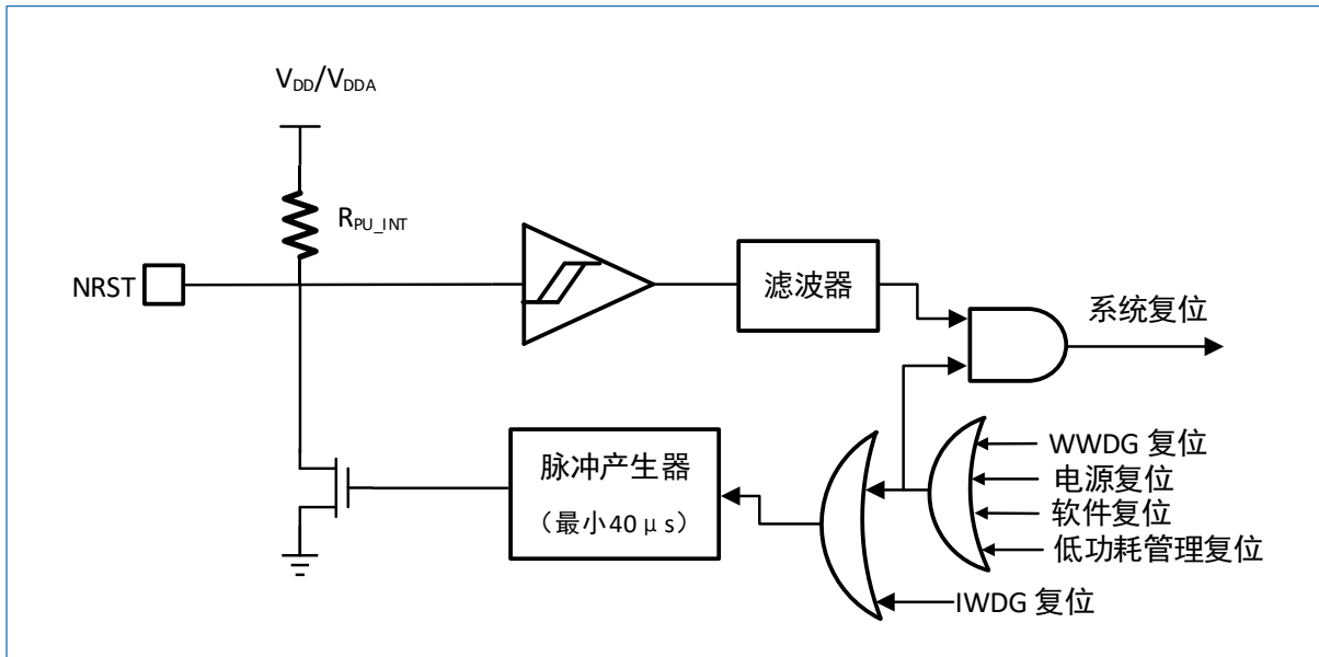
图 3-3 复位信号
