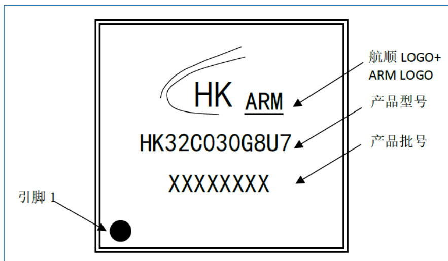
图 7-11 QFN28 丝印示例
