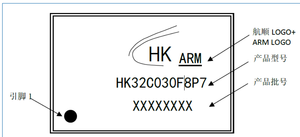
图 7-12 TSSOP20 丝印示例
