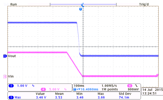
掉电响应： HT7333-1 ( I_{OUT}=250mA , T_{FALL}=100ms )
