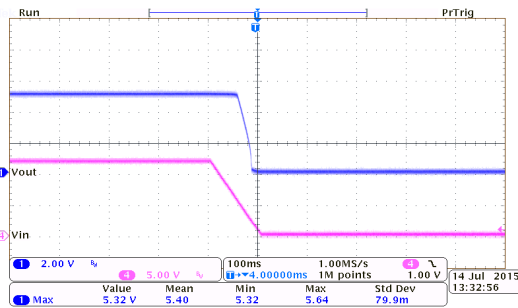
掉电响应： HT7350-1 ( I_{OUT}=250mA , T_{FALL}=100ms )
