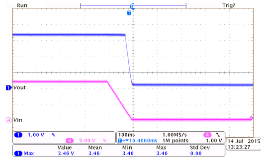
掉电响应： HT7333-1 ( I_{OUT}=0mA , T_{FALL}=100ms )
