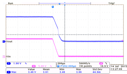
掉电响应： HT7333-1 ( I_{OUT}=250mA , T_{FALL}=0.1ms )
