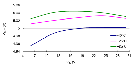
电压线性调整率: HT7350-1 ( I_{OUT}=10mA )
