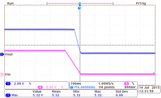
掉电响应： HT7350-1 ( I_{OUT}=0mA , T_{FALL}=100ms )
