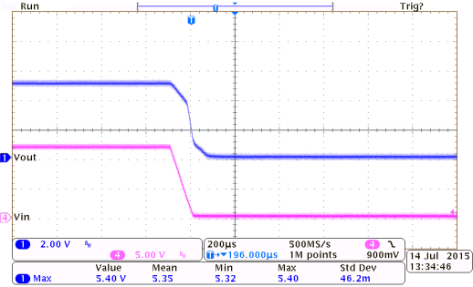
掉电响应： HT7350-1 ( I_{OUT}=250mA , T_{FALL}=0.1ms )
