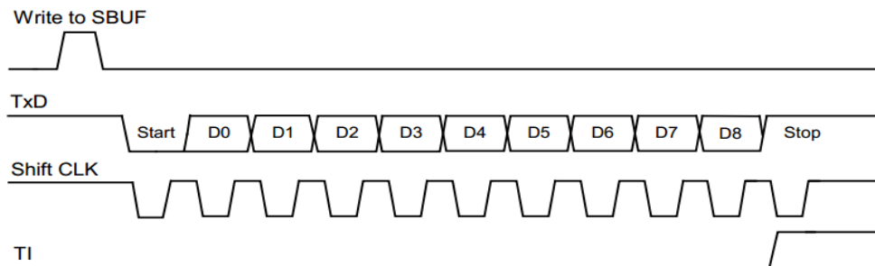
Figure 13-8 模式 2 数据发送时序框图
