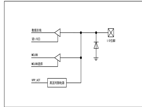
图1-4: PORTB5口的等效电路
