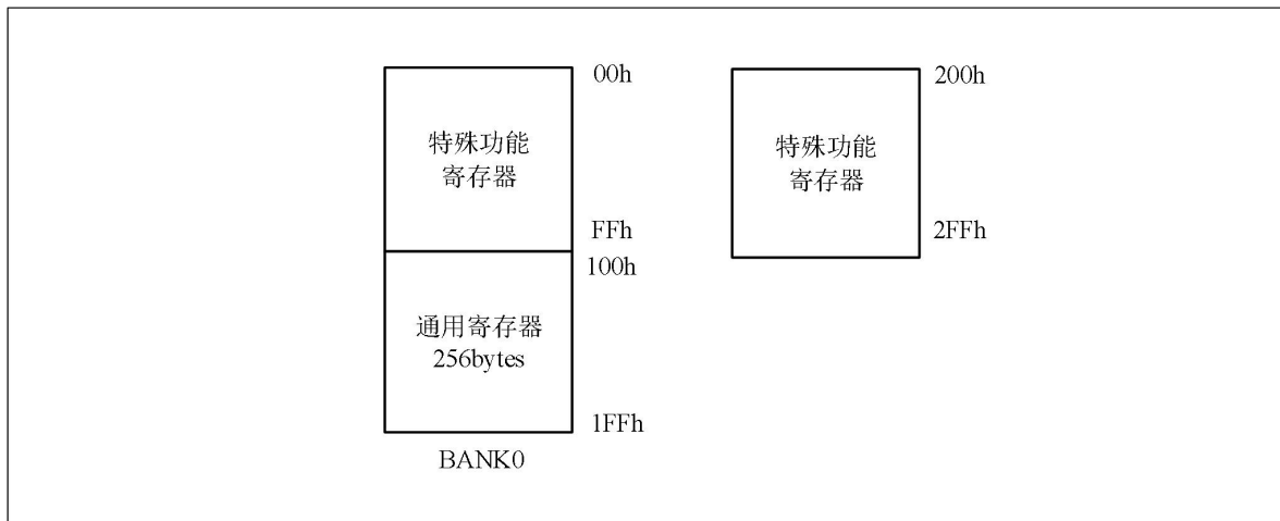
图2-2 数据存储映射
