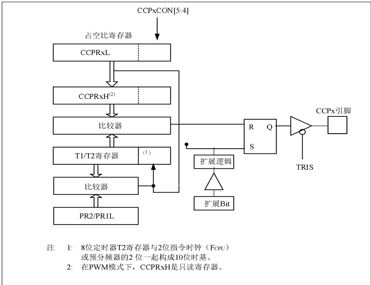
图8-7 PWM模式工作原理图
