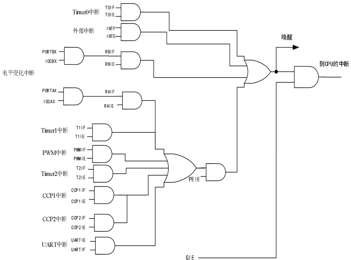
图6-1 中断示意图
