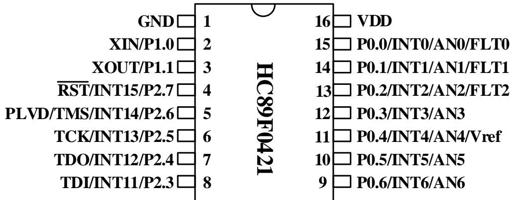
Figure 1-4 SOP16 引脚配置图
