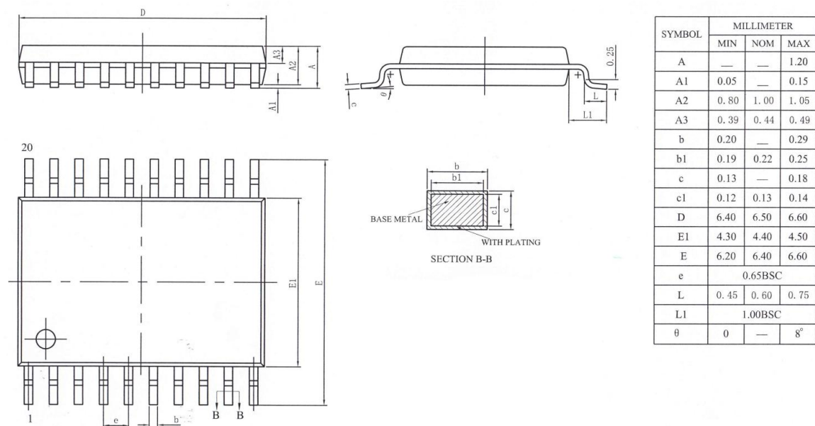
Figure 21-2 TSSOP20 封装尺寸
