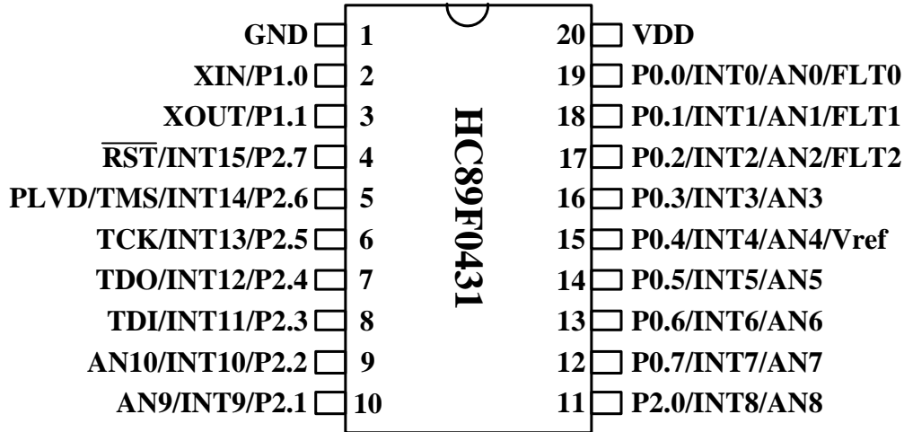
Figure 1-2 SOP20/TSSOP20 引脚配置图
