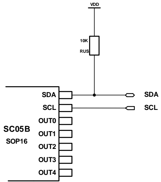
图3-5: I 2 C 查询方式
